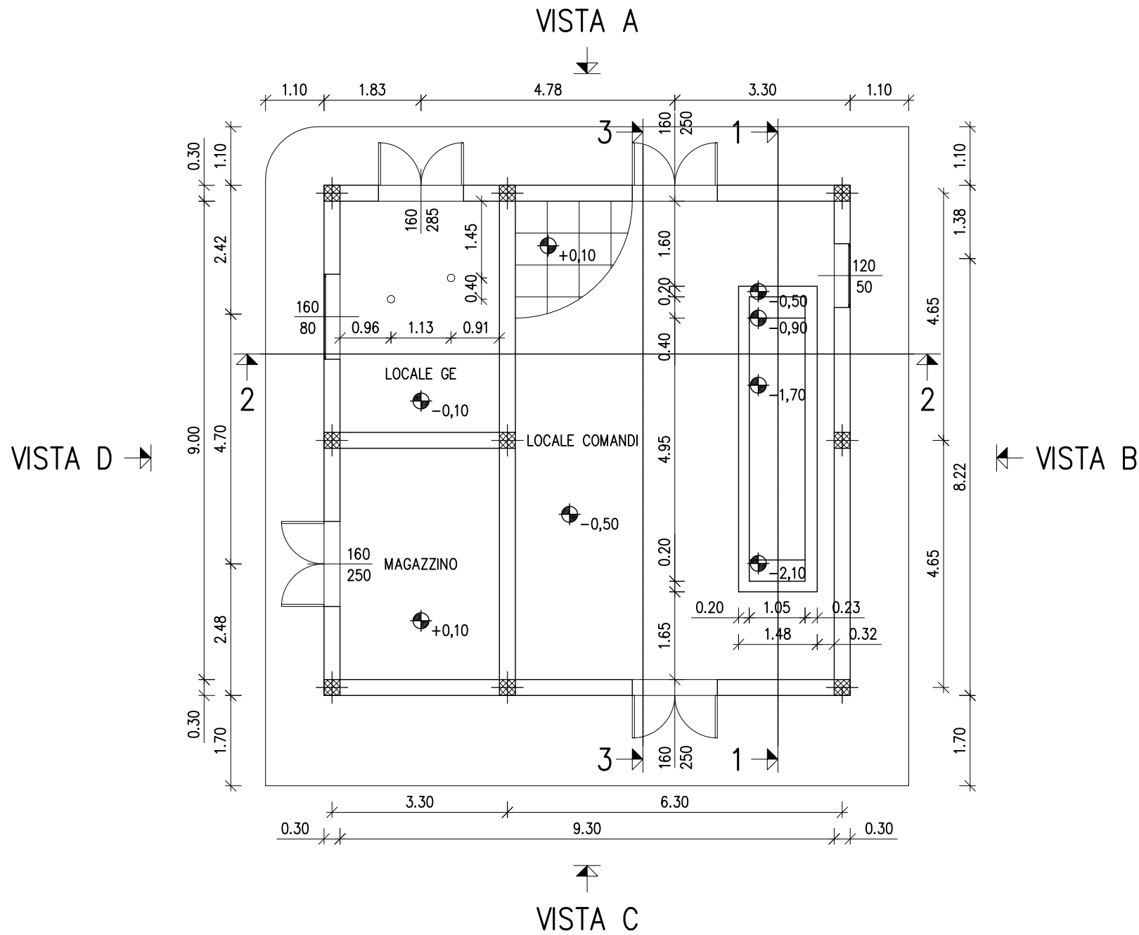
PLANIMETRIA
