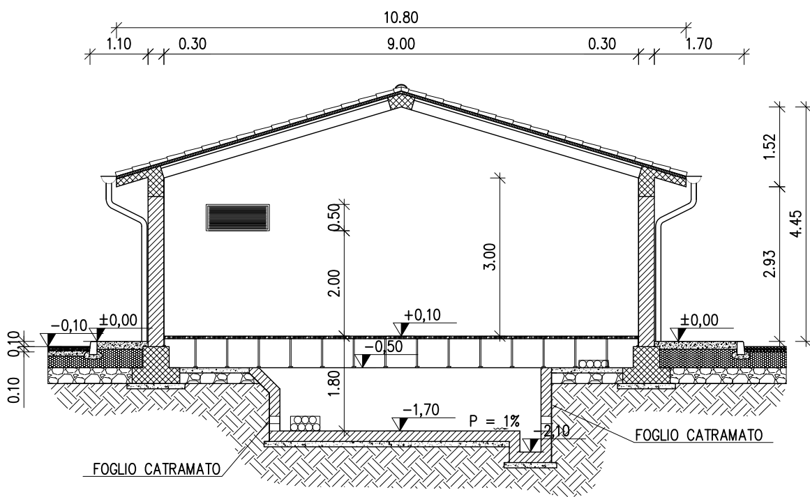
SEZIONE 1 - 1
