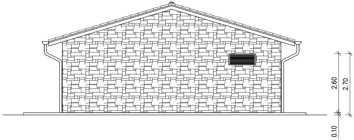
VISTA D
