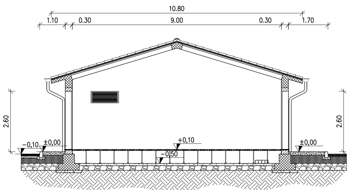
SEZIONE 3 - 3
