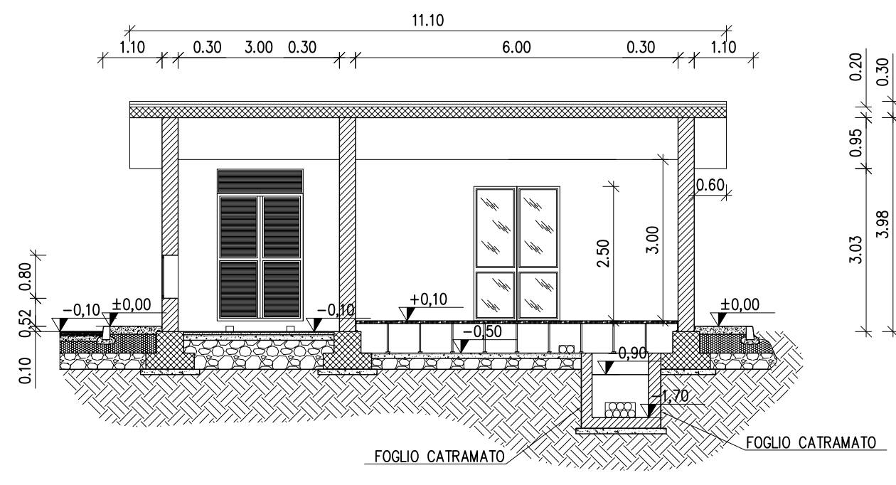
SEZIONE 2 - 2
